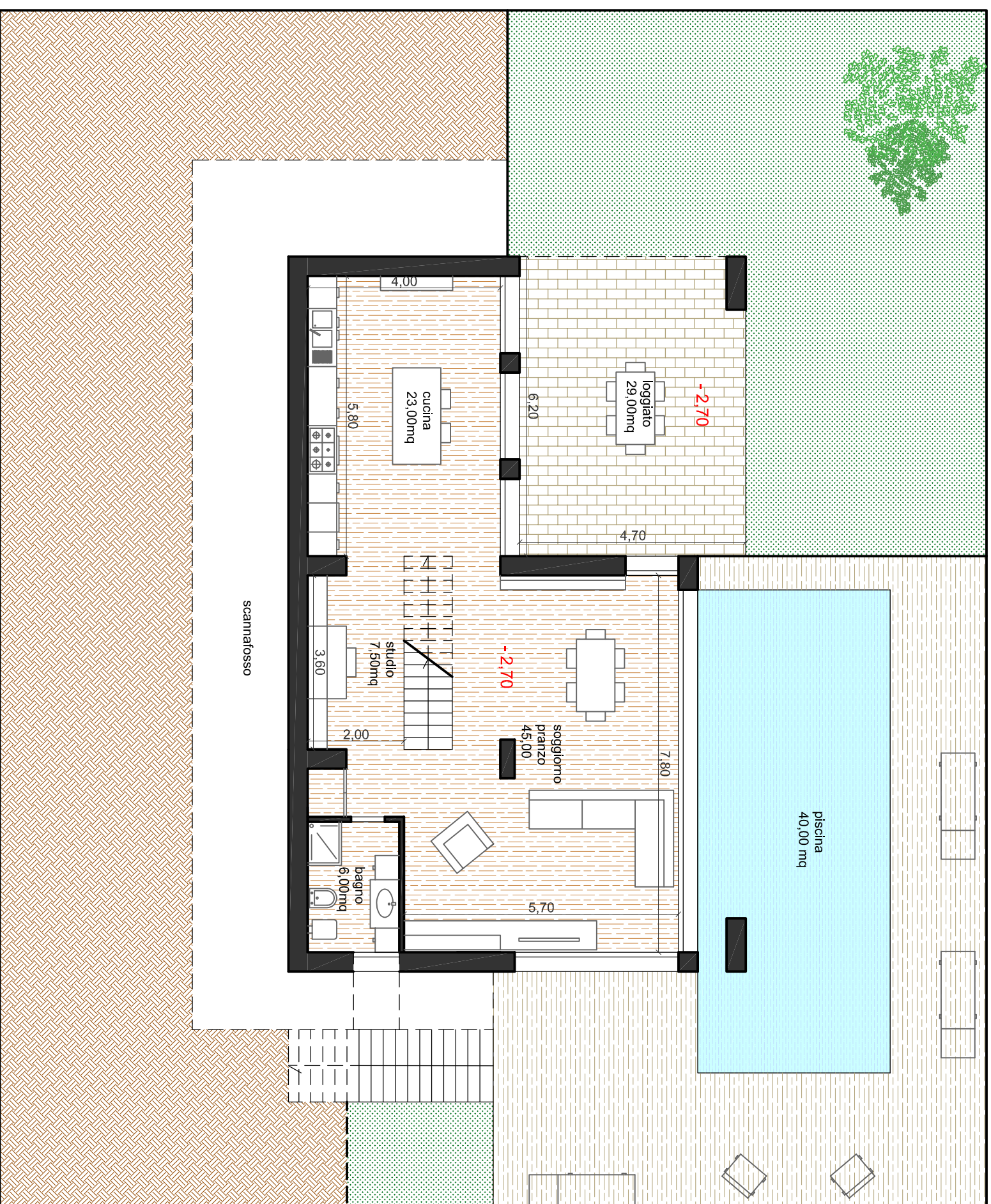
PIANO TERRA LIVELLO -1
